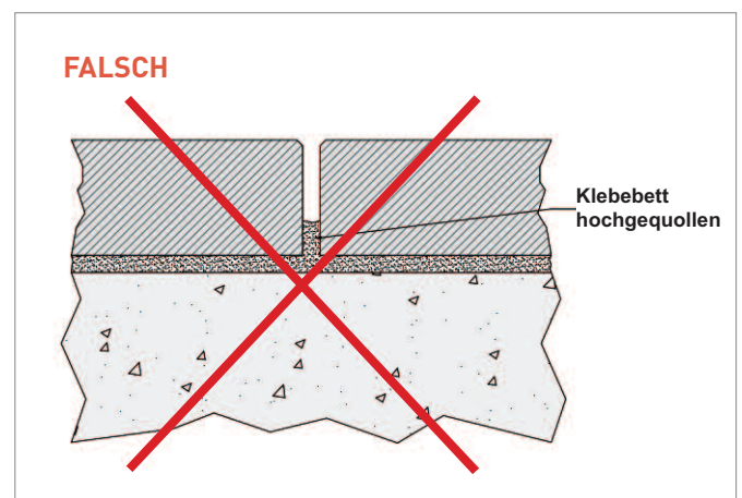
Abbildung 3: Klebebett hochgequollen = falsch!
