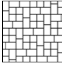
Mittelsteinverband Bedarf pro m 2 : 24/16/6 - 18,40 Stk. 16/16/6 - 9,20 Stk.
